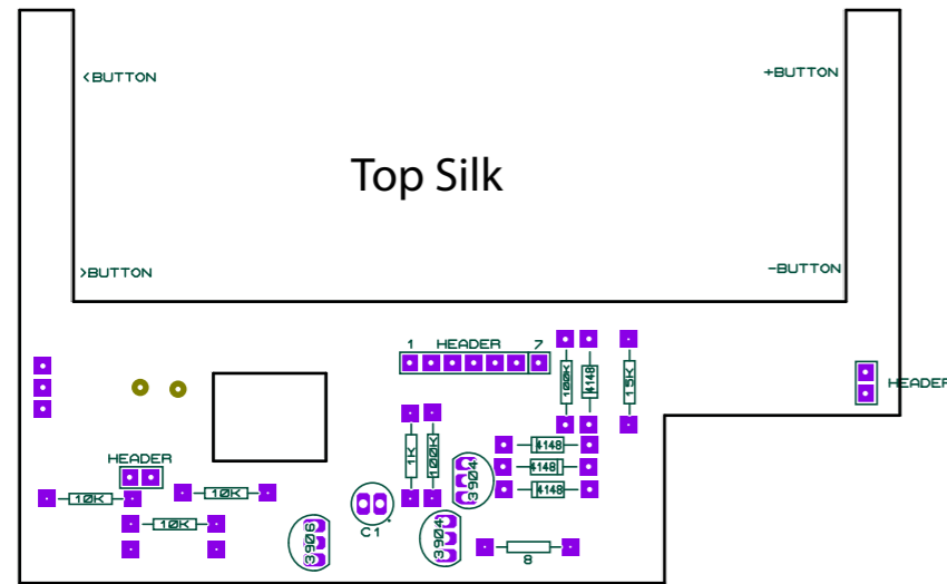
PCB Top
